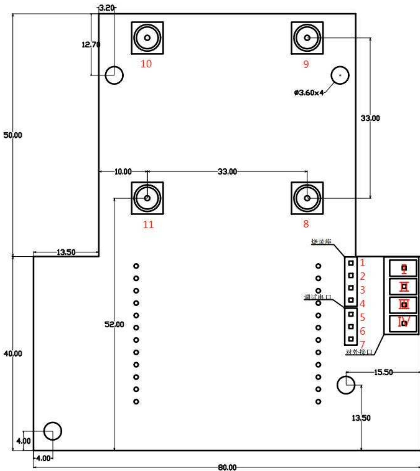
图4.1 PCBA尺寸图
